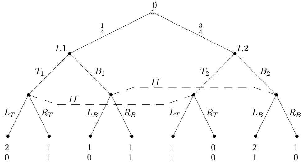
Figura 5.4: Un semplice gioco di segnalazione
